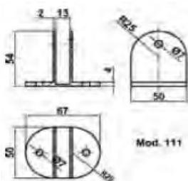
INOX DRŽAČI MODEL 111, 112, 113
