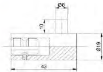
INOX VJEŠALICA MODEL 12
